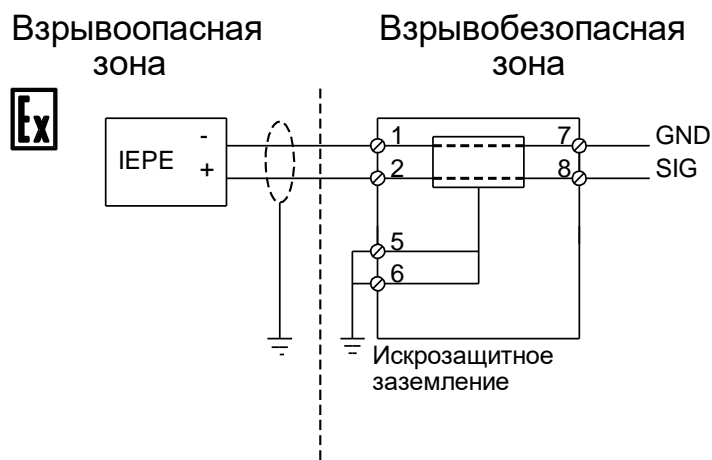
Рисунок 7 – Схема подключения барьеров безопасности ТИК-BIS.313.0X01
