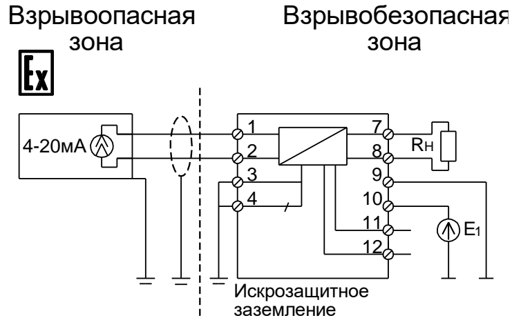
Рисунок 3 – Схема подключения барьеров безопасности ТИК-BIS.111.1X11 активный выход
