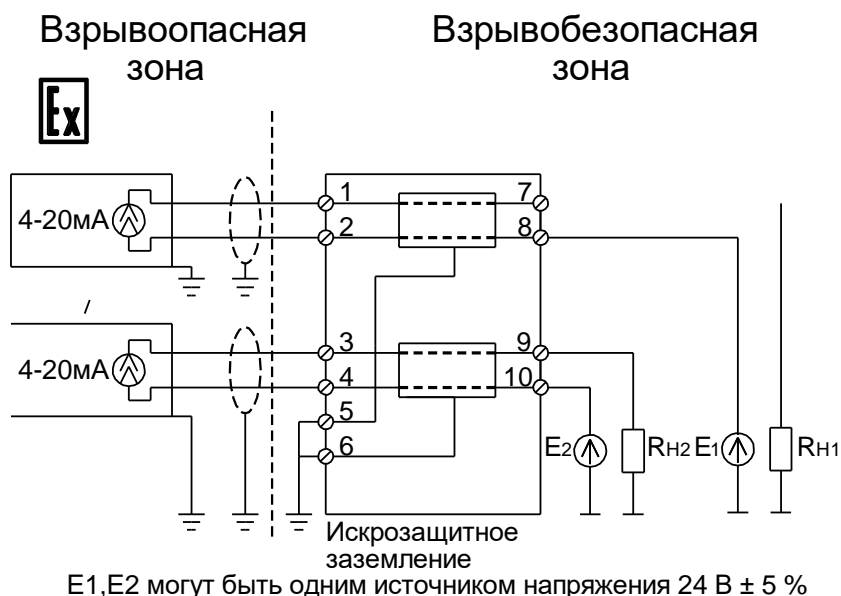
Рисунок 2 – Схема подключения барьеров безопасности ТИК-BIS.121.0X01
