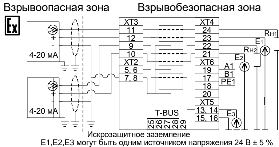
Рисунок 13 – Трехпроводная схема подключения барьера безопасности ТИК-BIS.527.1X02
