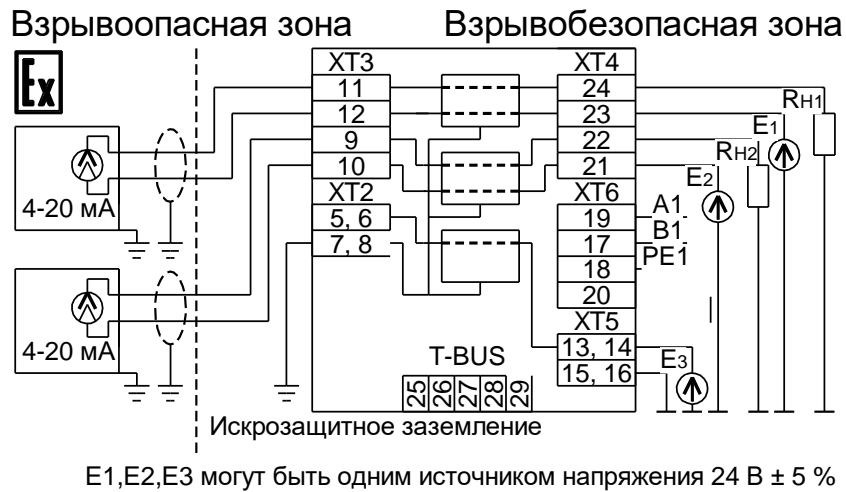
Рисунок 12 – Двухпроводная схема подключения барьера безопасности ТИК-BIS.527.1X02
