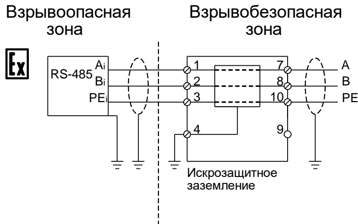
Рисунок 10 – Схема подключения барьеров безопасности ТИК-BIS.414.0X01
