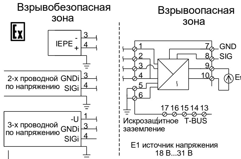
Рисунок 9 – Схема подключения барьеров безопасности ТИК-BIS.313.1X11
