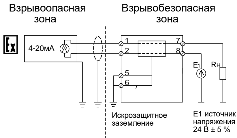
Рисунок 1 – Схема подключения барьеров безопасности ТИК-BIS.111.0X01
