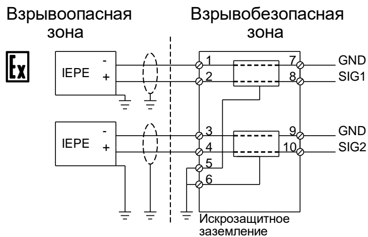
Рисунок 8 – Схема подключения барьеров безопасности ТИК-BIS.323.0X01
