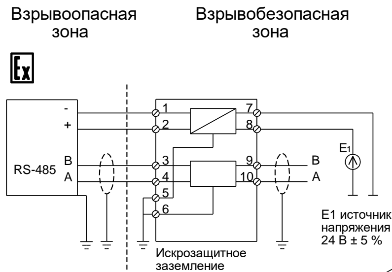
Рисунок 14 – Схема подключения барьеров безопасности ТИК-BIS.616.1X11
