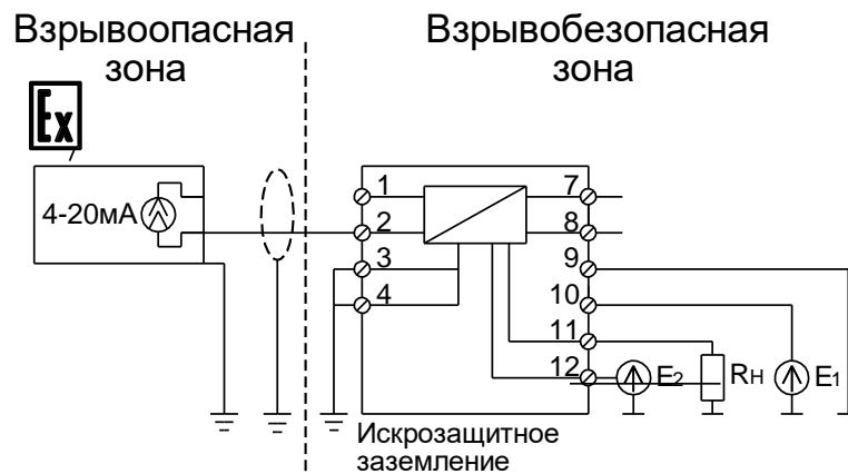
Рисунок 4 – Схема подключения барьеров безопасности ТИК-BIS.111.1X11 пассивный выход
