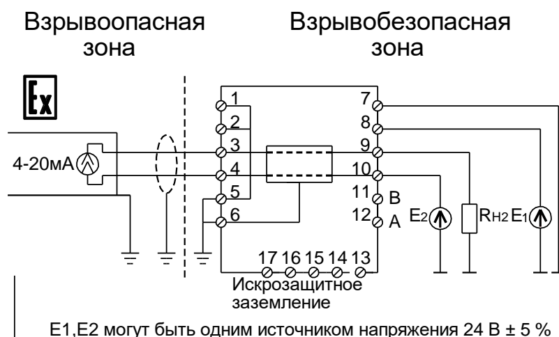
Рисунок 10 – Схема подключения барьера безопасности ТИК-BIS.517.1X01
