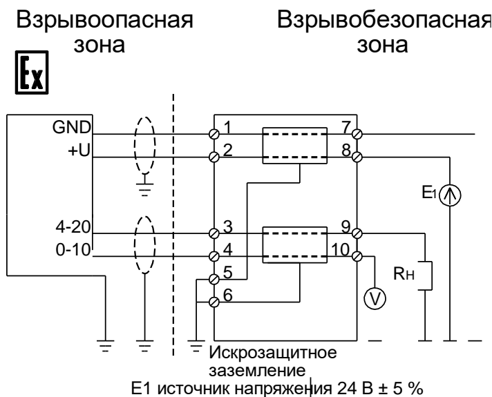
Рисунок 25 – Схема подключения барьеров безопасности ТИК-BIS.717.0X02
