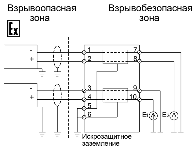
Рисунок 6 –Схема подключения барьеров безопасности ТИК-BIS.222.0X01
