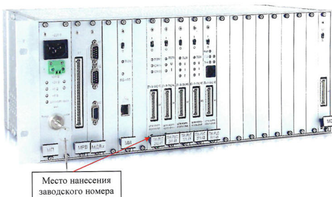
Рисунок 2 – Внешний вид аппаратуры ТИК-PLC в крейте
