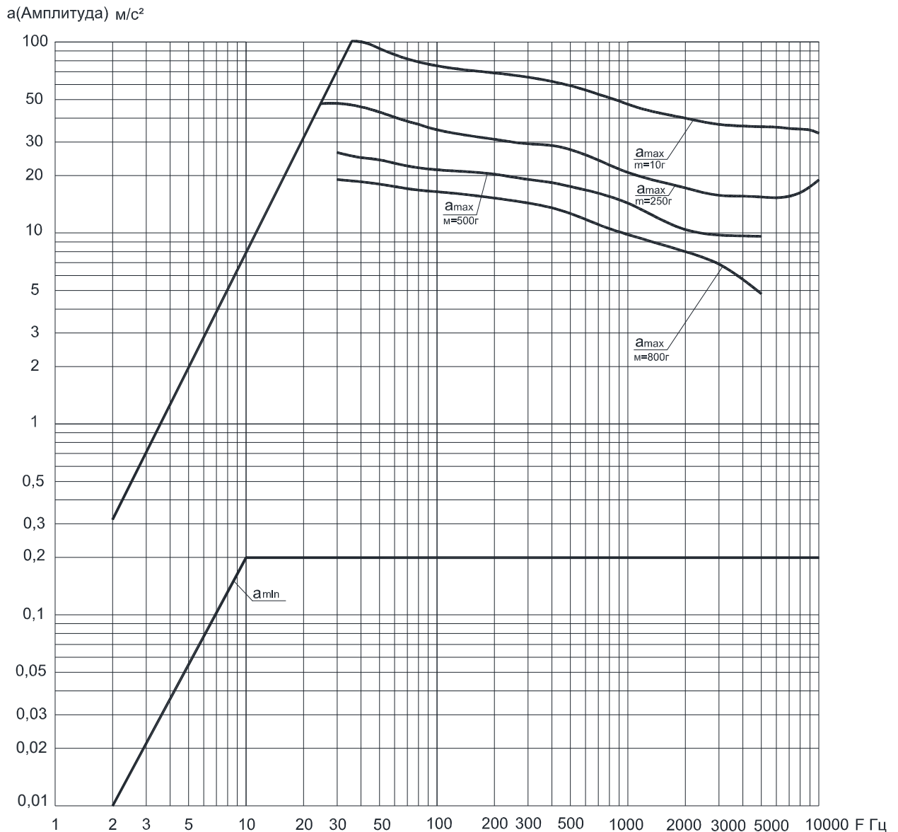
Рисунок 1 (а max – максимальные значения воспроизводимого ускорения для нагрузочных масс 10г, 250г, 500г, 800г; а min – минимальные значения воспроизводимого ускорения)
