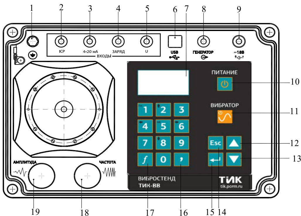
Рисунок 4 Панель вибростенда
